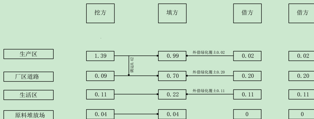
图 2.4-1 土石方流向图 单位：万 m 3
